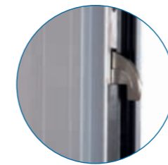
SERRURE 5 POINTS : 4 COFFRES DE PÊNE RÉPARTIS SUR LA HAUTEUR DE LA PORTE
